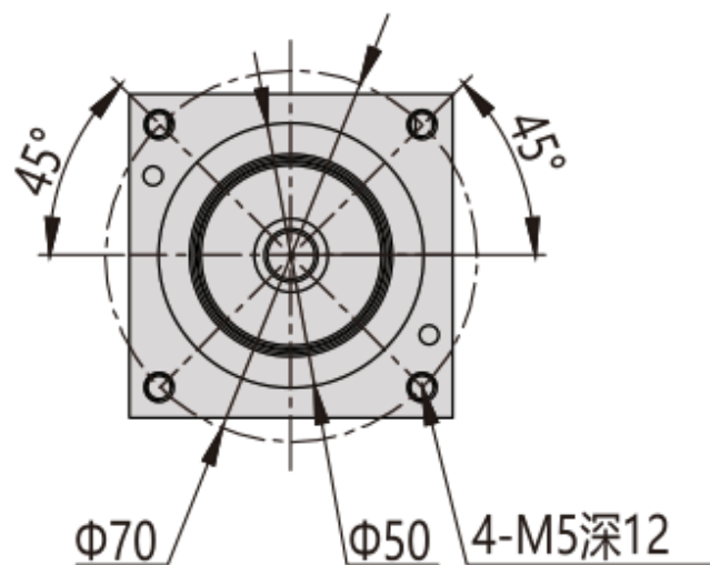
安装电机尺寸图
