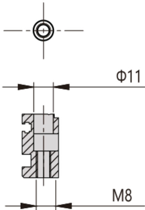
B向视图(1:1)
