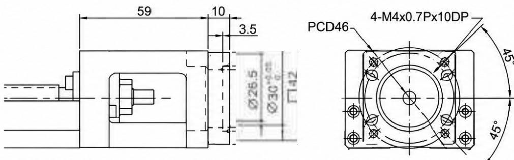
Motor Adaptor Flange F1
