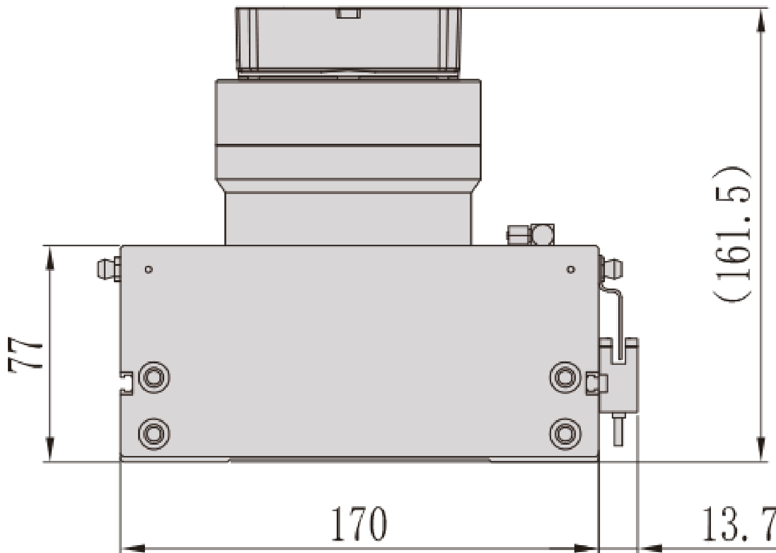
MS17 · Dustproof type · view 3
