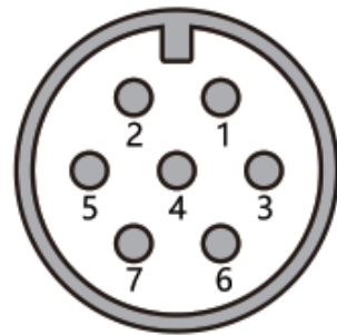
传感器航插接线图
