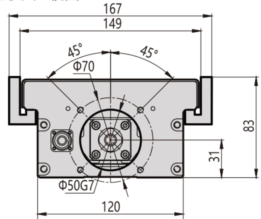
电机法兰视图
